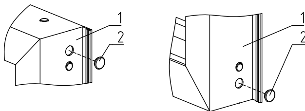
Рис. 11. Установка заглушек PP12:
