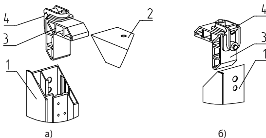
Рис. 2. Установка соединителей:
