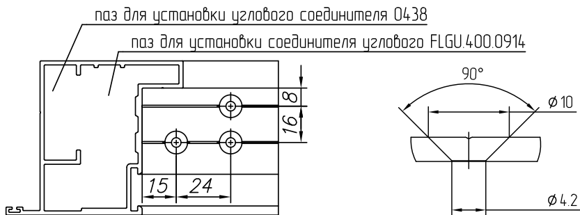
Рис. 5. Изготовление отверстий:
